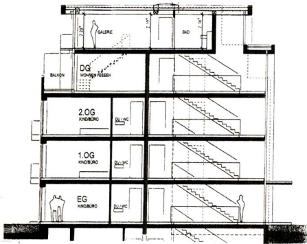
Schnitt Haus F - G - H
