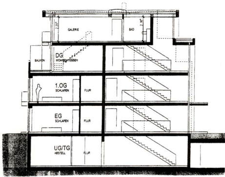
Schnitt Haus A bis E
